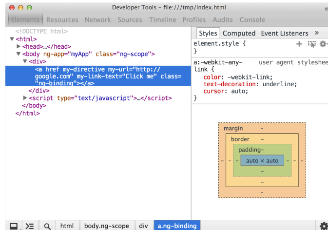
Updating template
